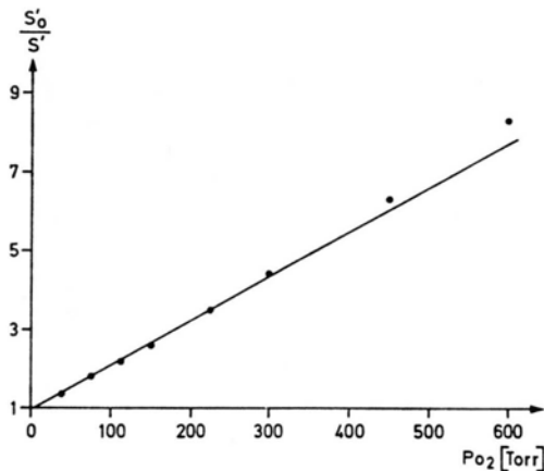
Abb. 3. Eichkurve der p\text{O}_2 -Optode. ( S' = Fluoreszenzintensität in Abhängigkeit vom Sauerstoffdruck; S'_0 = S' bei einem p\text{O}_2 von 0 Torr; \lambda(\text{excitation}) = 342 \text{ nm} ; \lambda(\text{emission}) = 395 \text{ nm} .)
